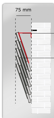
Supporto verticale Systembox
