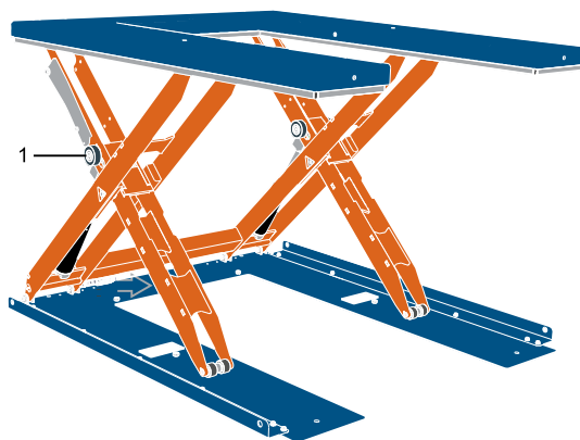
Figura 12 Punti di lubrificazione
