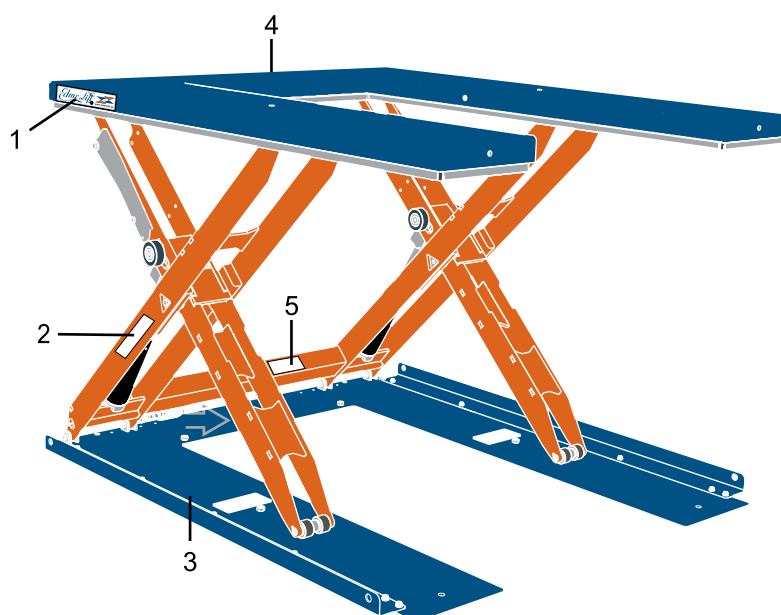
Figura 22 Etichette e cartelli
