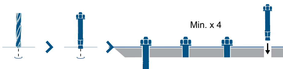
Figura 18 Ancorare la piattaforma elevatrice alla base impiegando almeno quattro bulloni a espansione.
