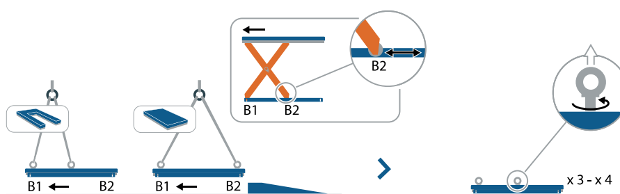
Figura 15 Ubicazione della piattaforma elevatrice
